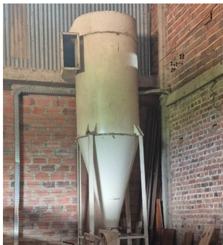
51. CICLONE
